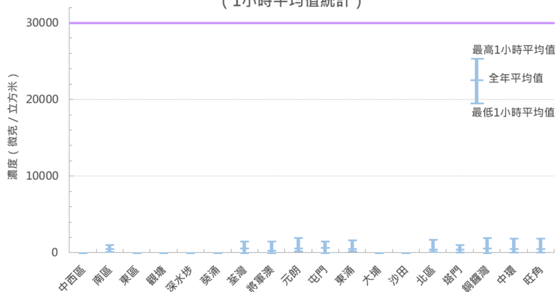
圖 7a：2024年一氧化碳水平的監測結果 (1小時平均值統計)
