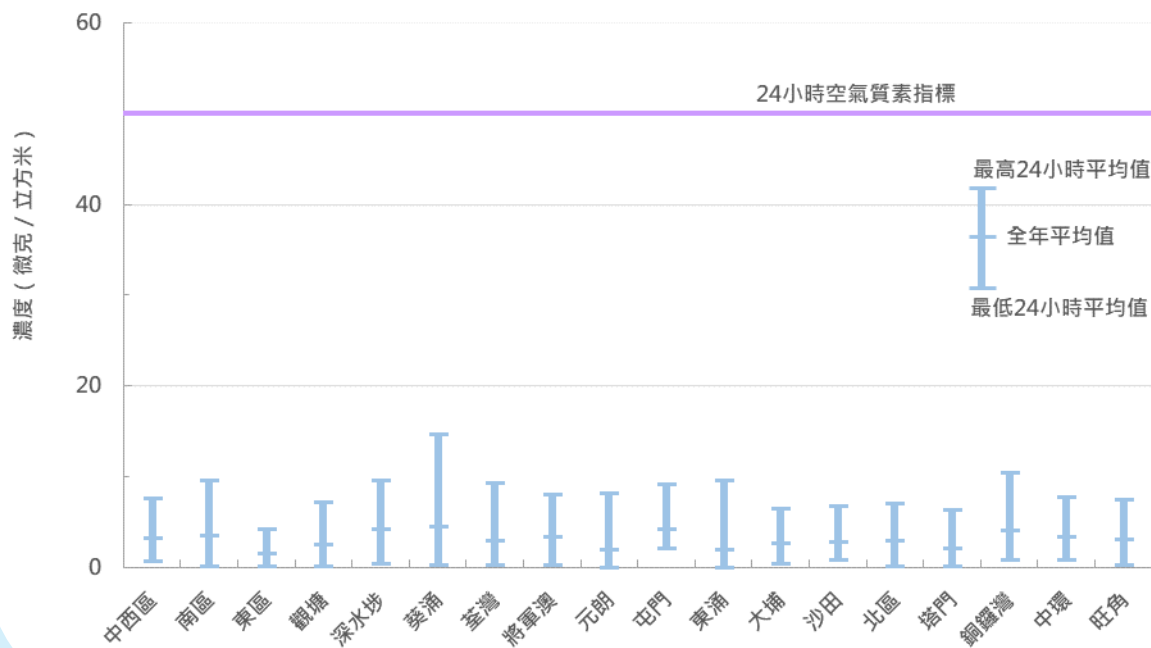
圖 2b : 2024年二氧化硫水平的監測結果 ( 24小時平均值統計 )
