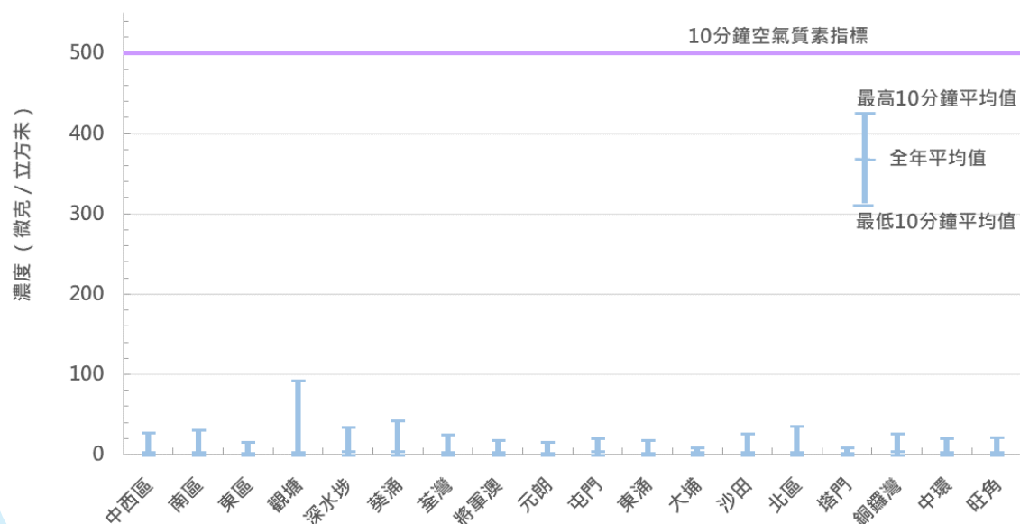
圖 2a : 2024年二氧化硫水平的監測結果 ( 10分鐘平均值統計 )
