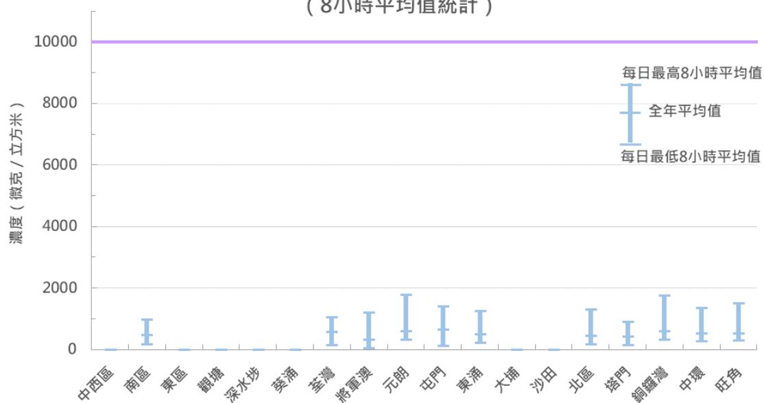
圖 7b：2024年一氧化碳水平的監測結果 (8小時平均值統計)
